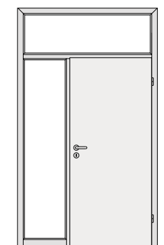
Élément pare-vent avec une partie latérale et imposte vitrée
